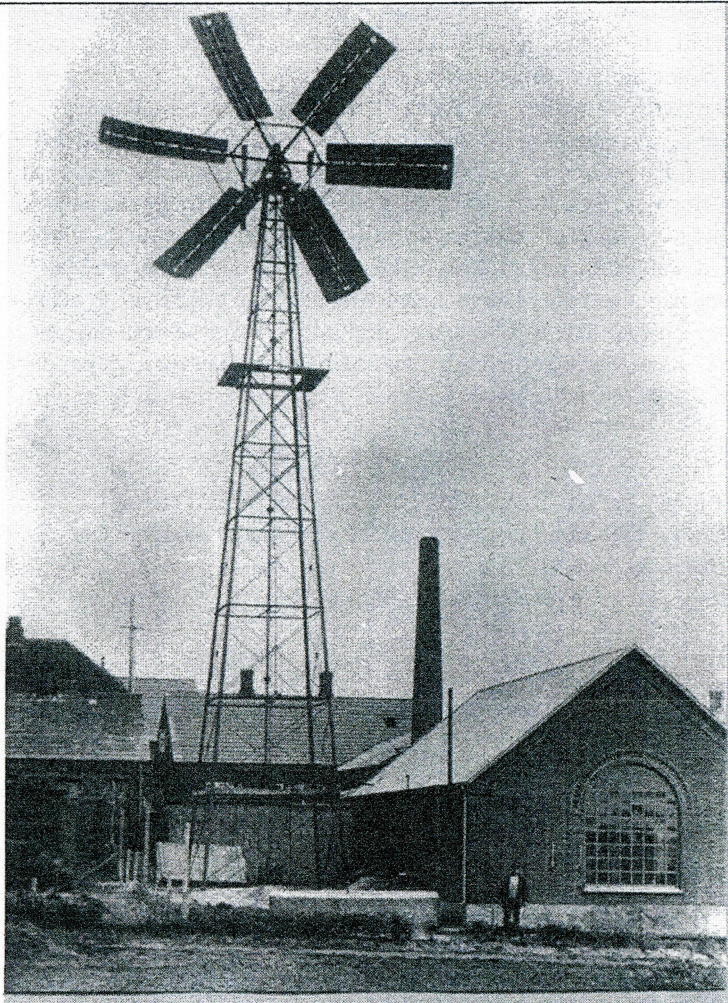
Elektricitetsværkets Vindmølle
